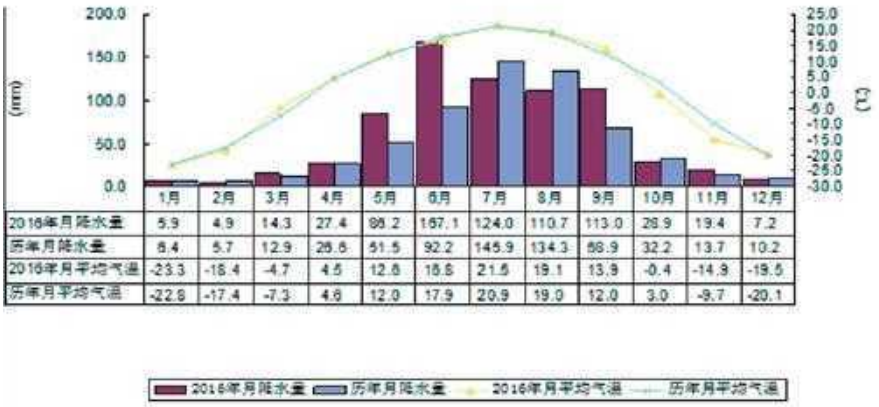
图 1 2016 年伊春市平均气温、降水量逐月演变图
