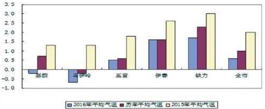
图 2 2016 年与历年、2015 年伊春市平均气温比较图
