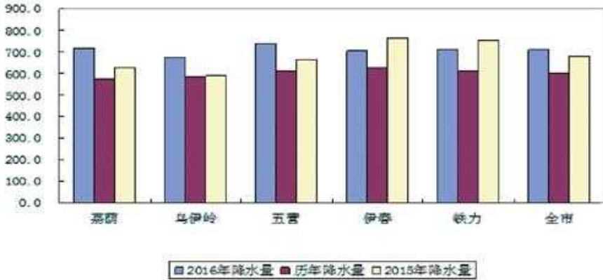
图 3 2016 年与历年、2015 年伊春市降水量比较图
