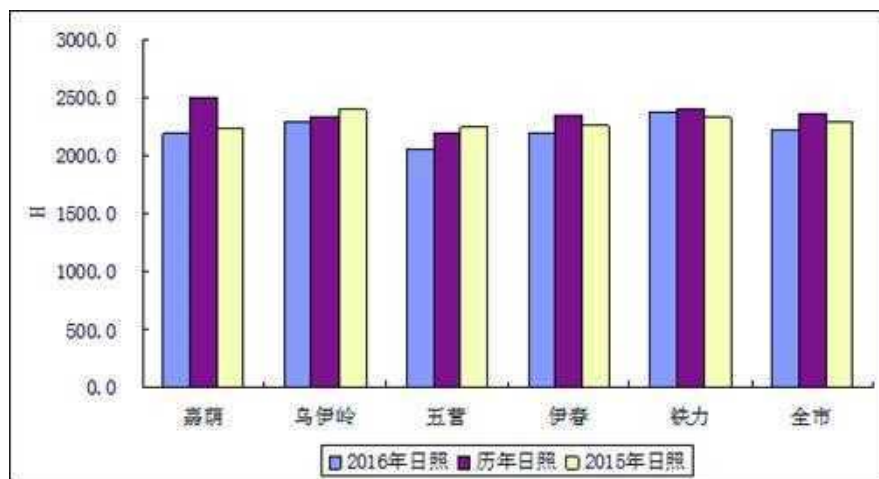
图4 2016年与历年、2015年伊春市日照时数比较图
